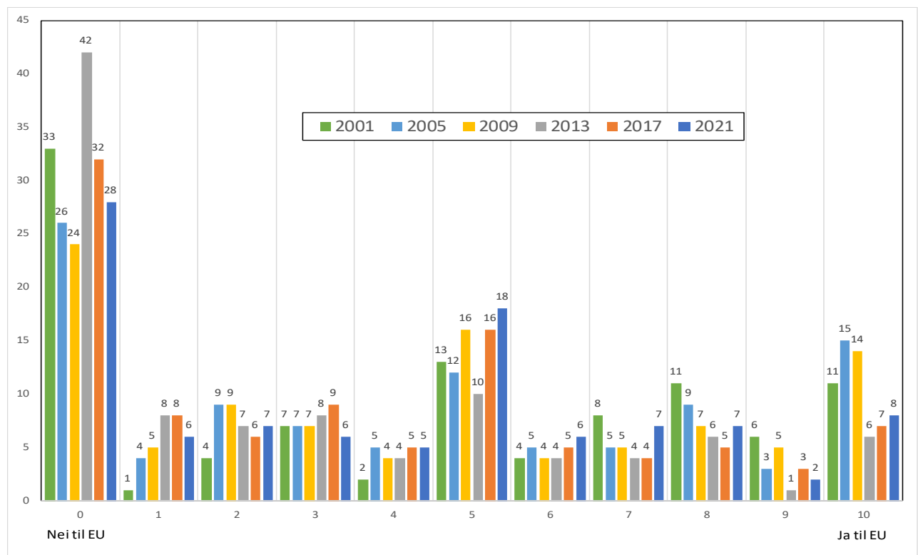
Figur 1. Holdning til norsk EU-medlemskap blant dem som er mest positive til miljøvern. 2001-2017.
