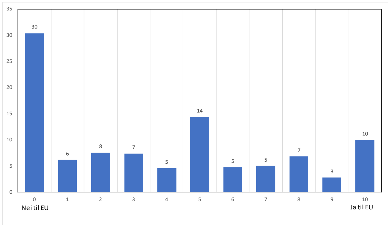
Figur 2. Holdning til norsk EU-medlemskap blant dem som er mest positive til miljøvern. Gjennomsnitt 2001-2021.
